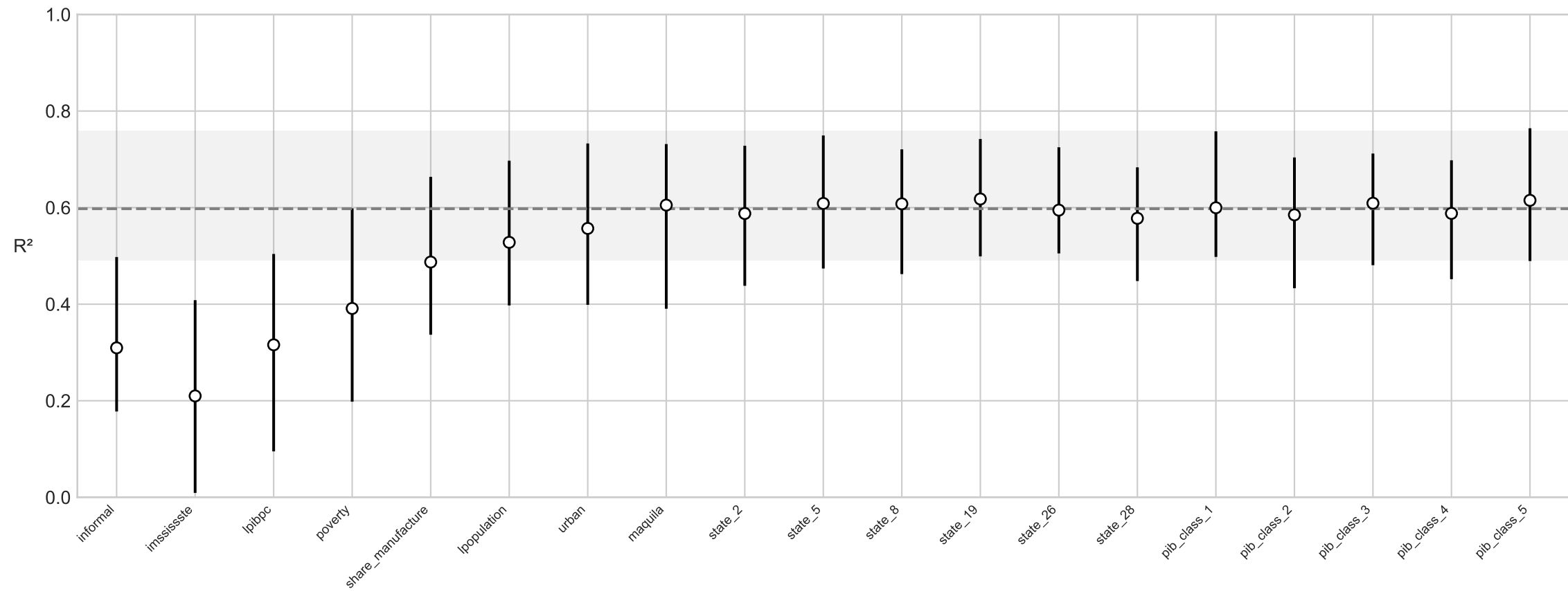
V4a: Importancia de variables — PS nuisance (BART Probit)
