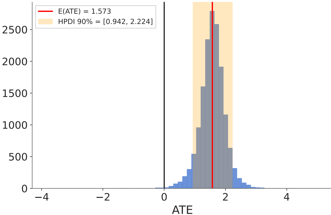
Distribución inducida del ATE AIPW + PS Probit-BART (muestra recortada)
