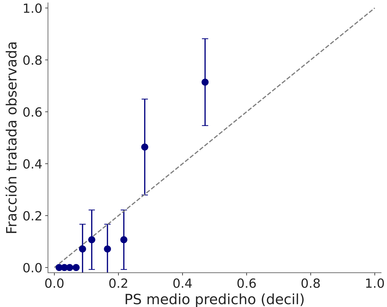
Calibración — BART
