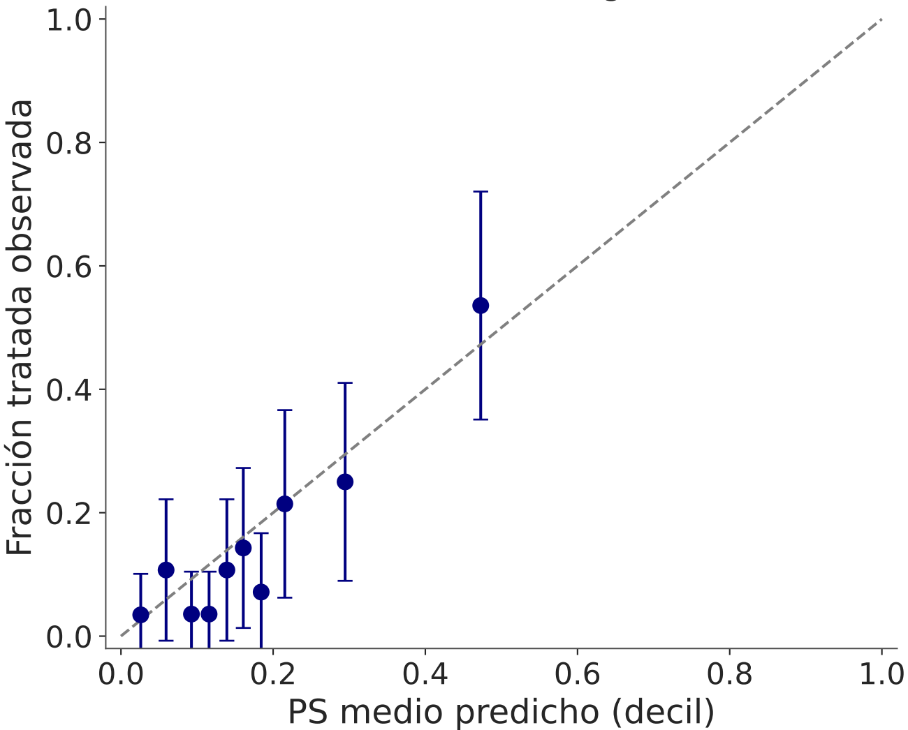
Calibración — Logit
