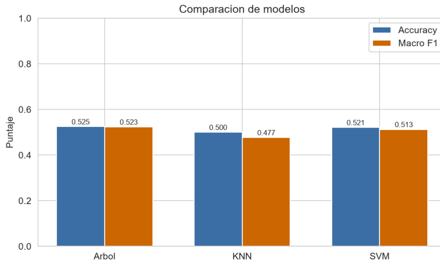
Figura 7: Comparación de exactitud y Macro F1 de los tres modelos.
