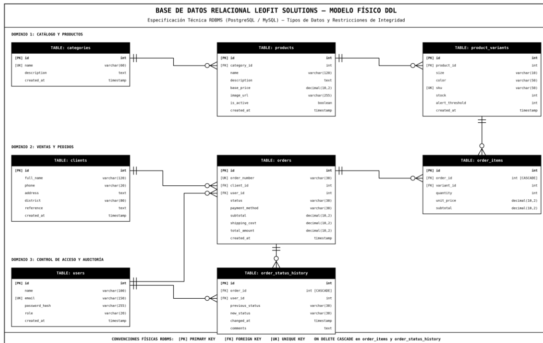
Figura 11: Diagrama de Modelo Físico DDL (PostgreSQL) Normalizado BCNF.
