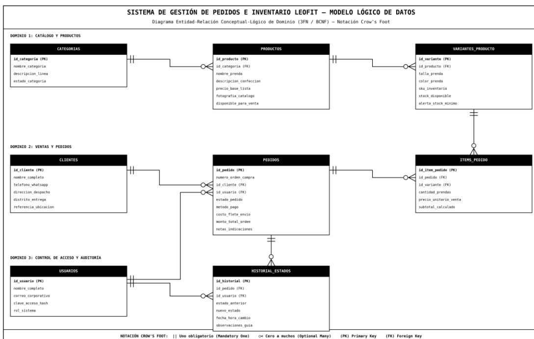
Figura 10: Diagrama de Modelo Lógico Relacional (3FN) de LeoFit Solutions.
