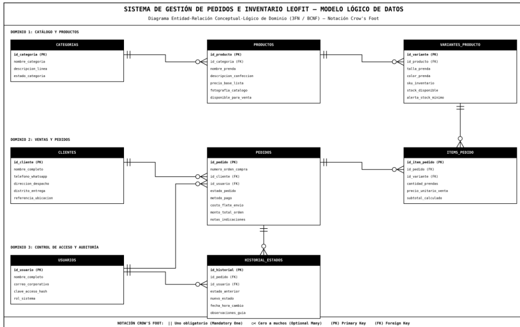
Figura 8.1: Modelo Entidad-Relación Lógico de Base de Datos
