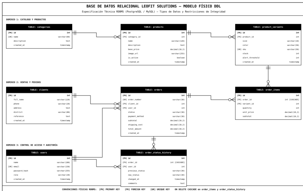
Figura 8.2: Modelo Físico Relacional DDL de Base de Datos
