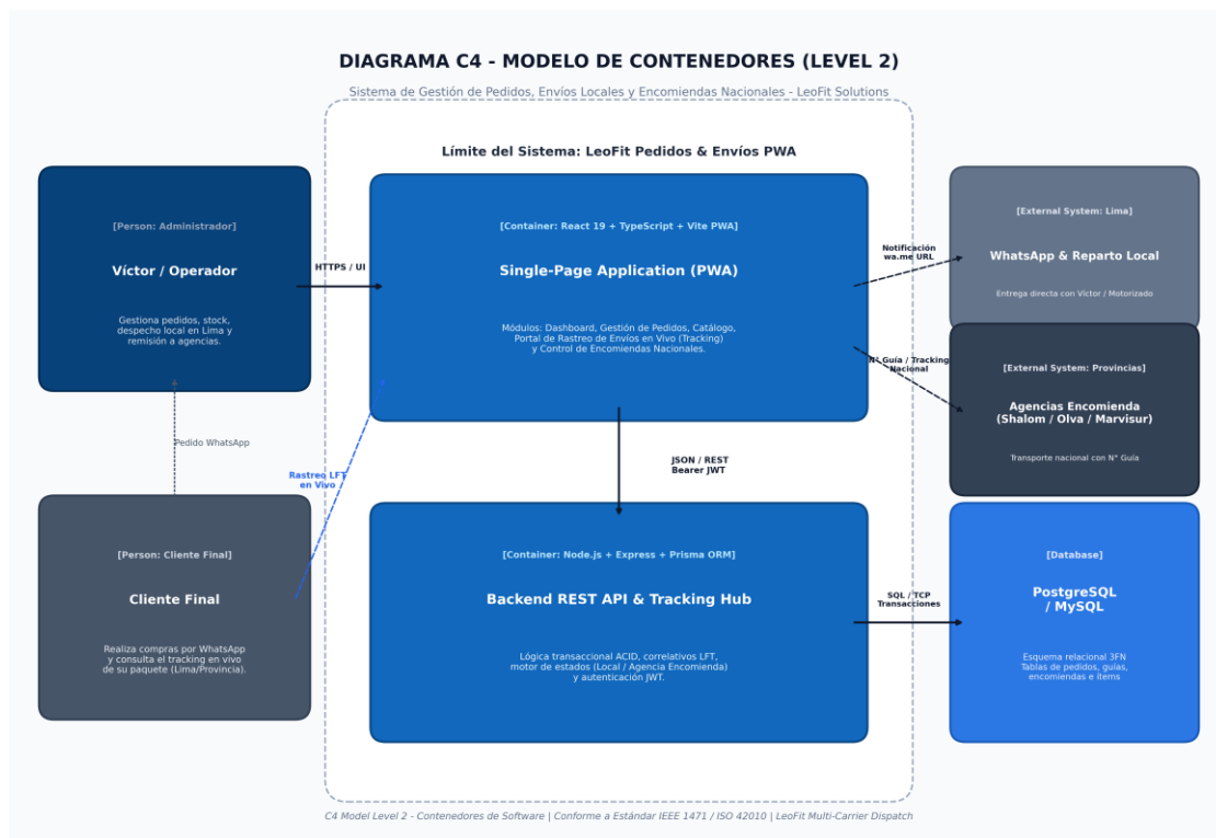
Figura 7.1: Arquitectura General del Sistema - Modelo C4
