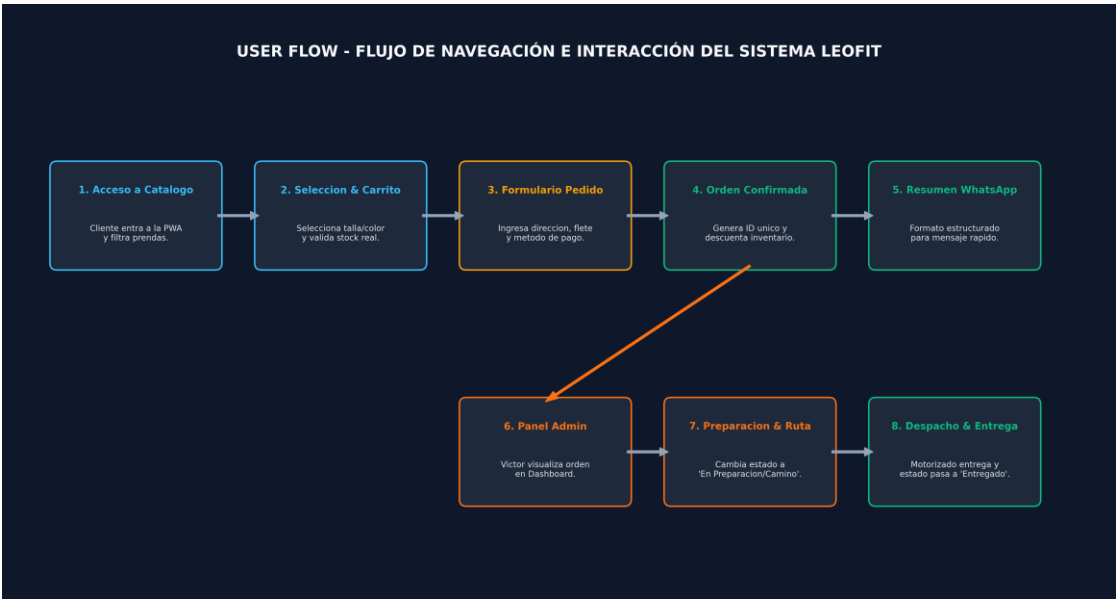
Figura 4.2: Diagrama de Flujo de Navegación del Usuario (User Flow)
