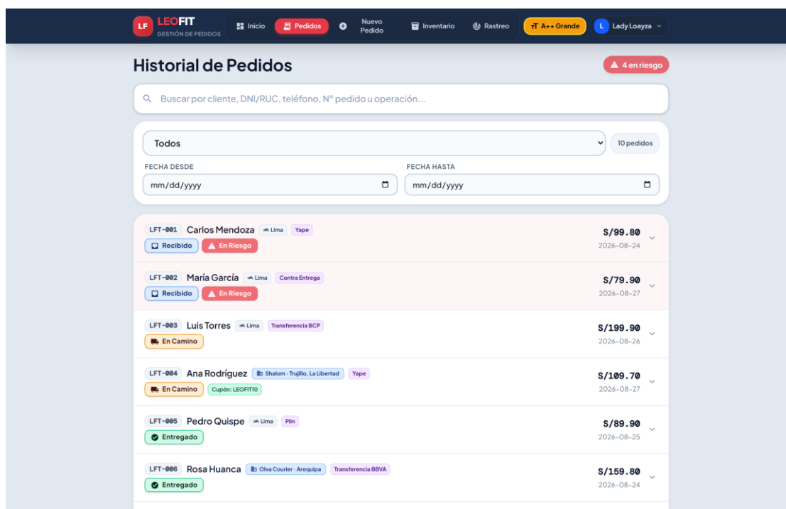
Figura 6: Bandeja Centralizada de Gestión de Pedidos con Filtros por Estado
