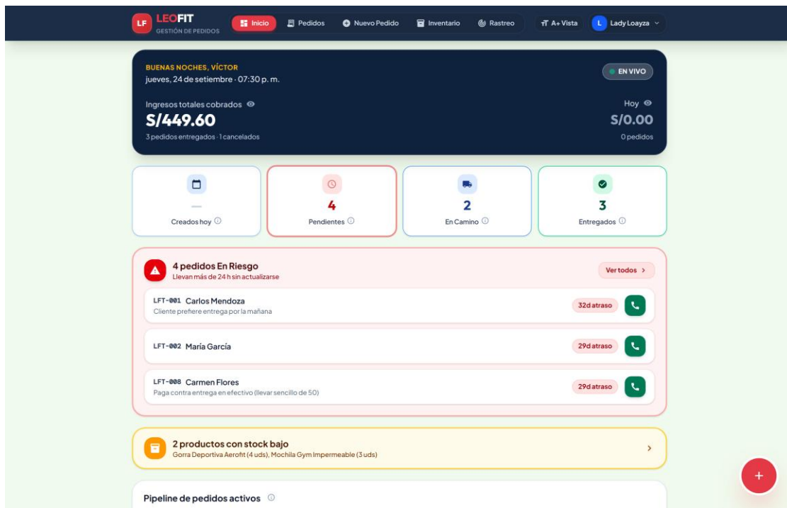
Figura 2: Dashboard Operativo con Tarjetas Métricas y Pipeline en Tiempo Real
