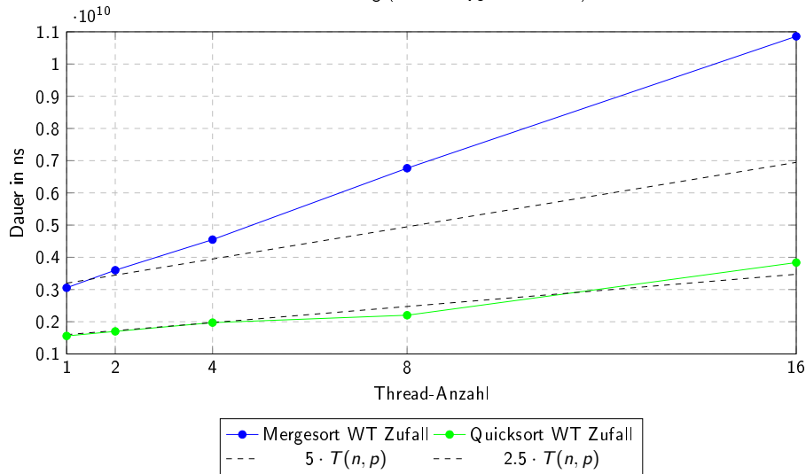
Abbildung: Weak Scaling (Worker-Thread): Die gestrichelten Linien zeigen die theoretisch zu erwartenden Laufzeitverbesserungen. WT = Worker-Thread-Variante
