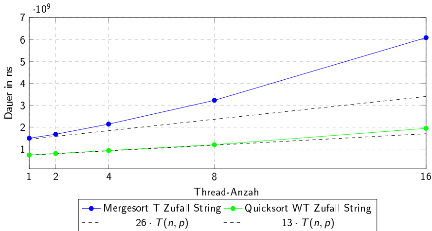
Abbildung: Weak Scaling (String): Die gestrichelten Linien zeigen die theoretisch zu erwartenden Laufzeitverbesserungen. T = Tiefenbasierte Thread-Erzeugung, WT = Worker-Thread-Variante
