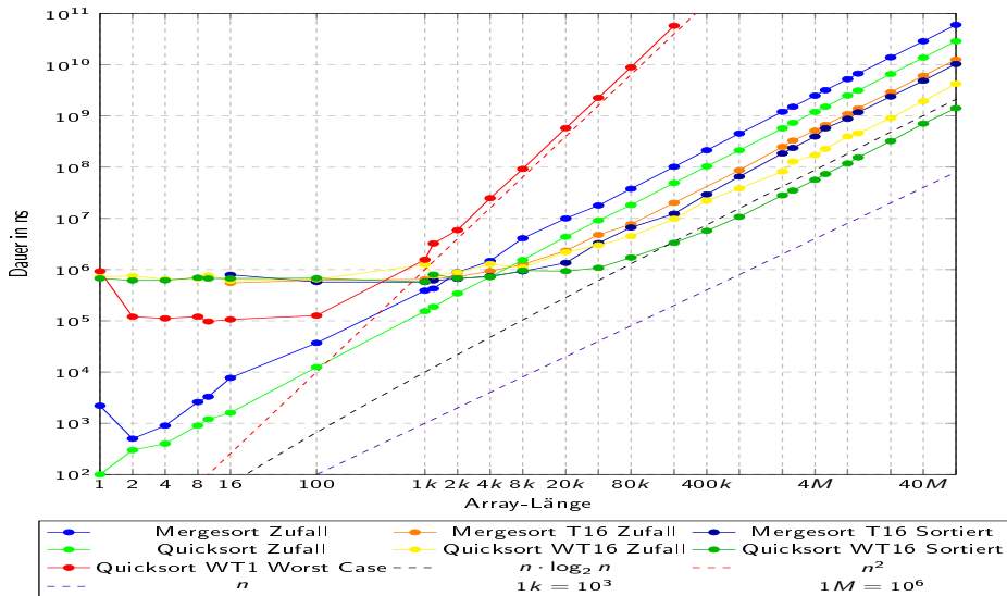
Abbildung: T16 = Tiefenbasierte Thread-Erzeugung mit 16 Threads. WT16 = Worker-Thread-Variante mit 16 Worker-Threads
