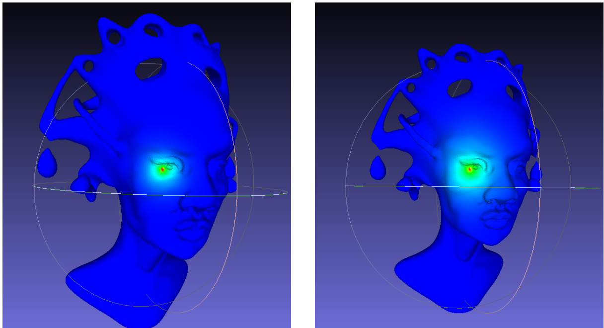
FIGURE 5 – Valeur de la température sous forme de heatmap pour une source de 100 degrés : après 2000 itérations (à gauche) et après 10000 itérations (à droite).
