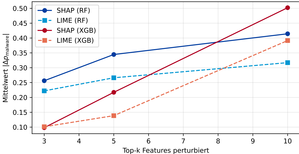
Fidelity: SHAP vs. LIME für zwei baumbasierte Klassifikatoren
