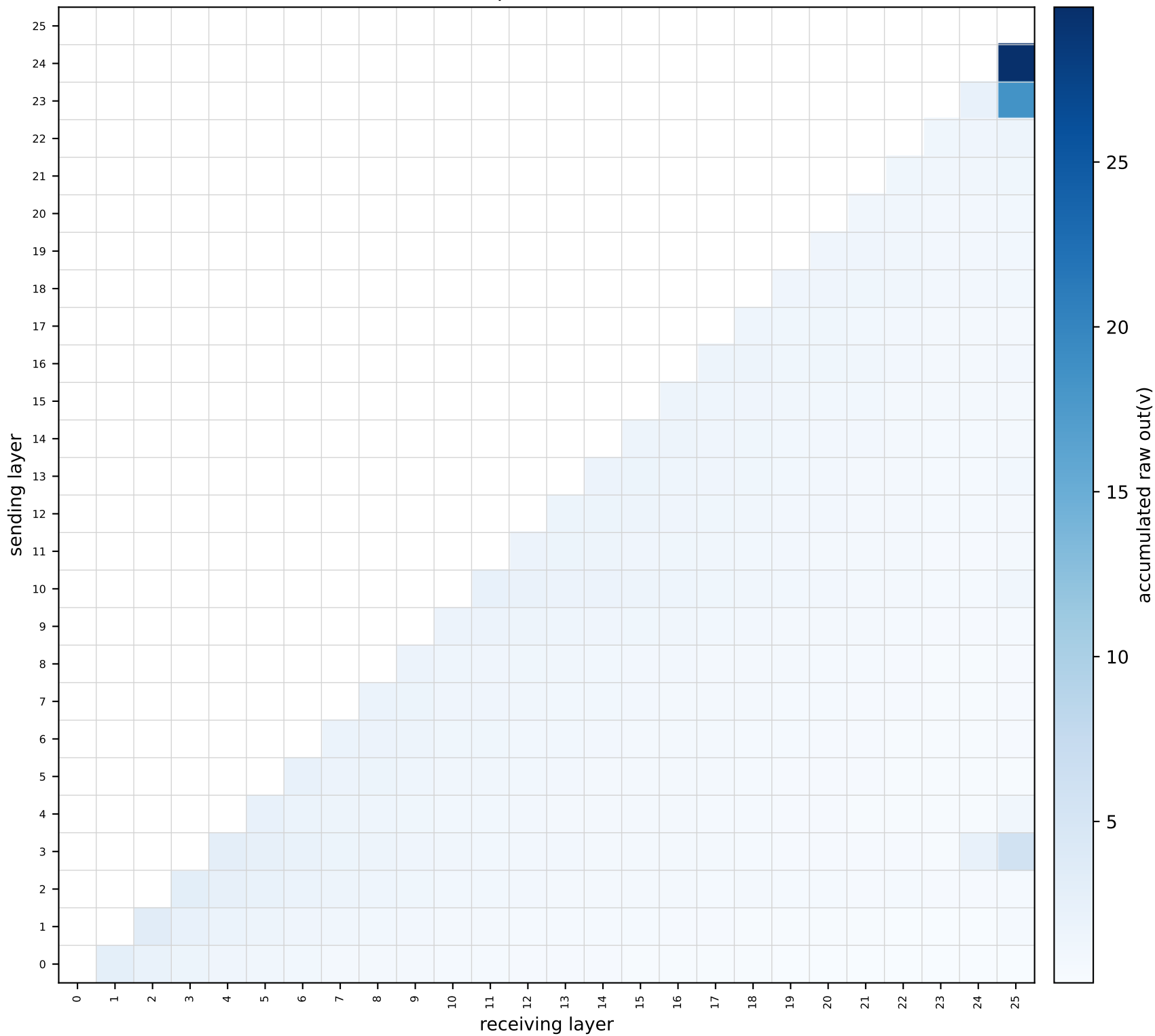
deepseek-v2-lite
