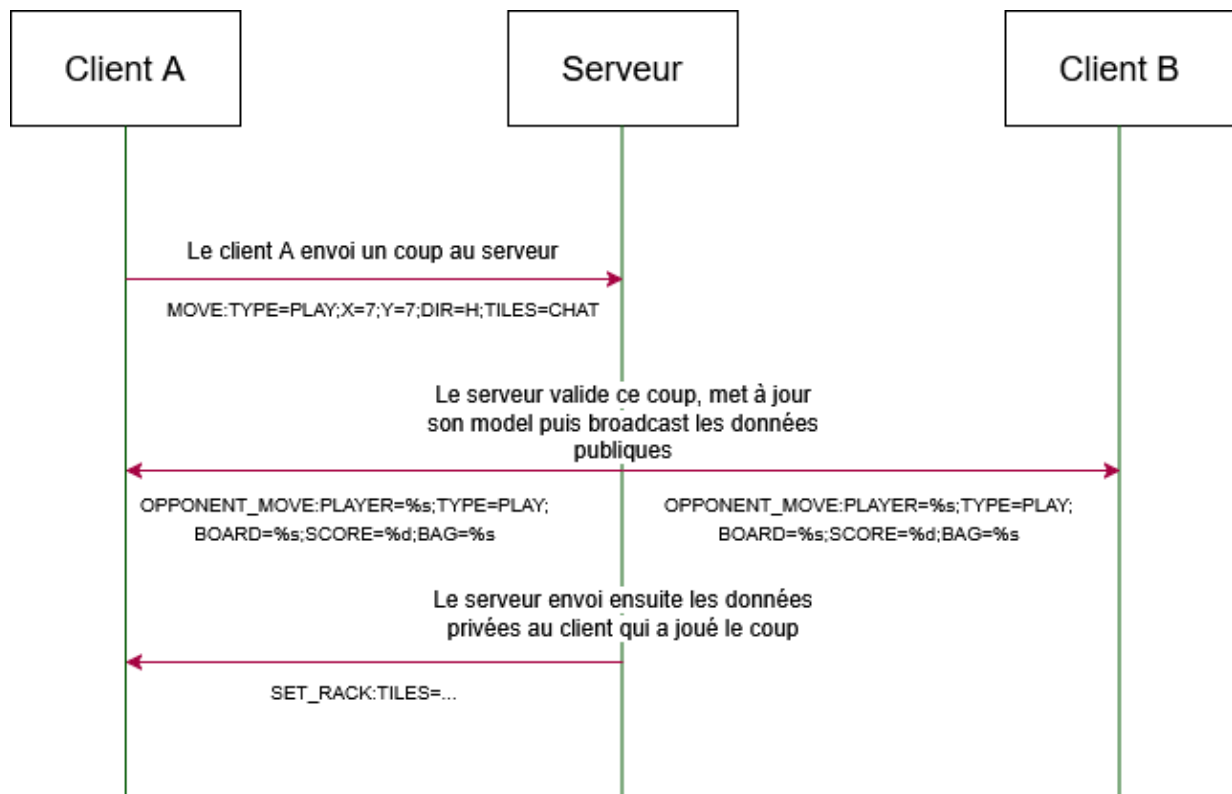
FIGURE 9 – Flux d'un coup valide dans une partie à deux clients (F39)
