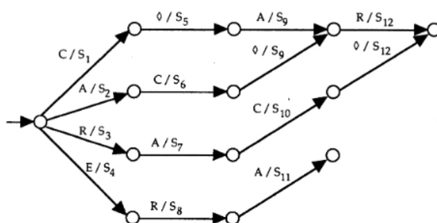
FIGURE 6 – Graphe du GADDAG semi-minimisé pour « CARE ». (Source : [6])
