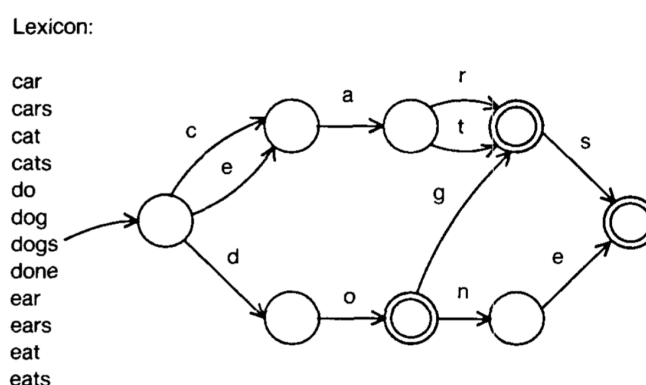
FIGURE 5 – Exemple d’une structure DAWG. (Source : [1])
