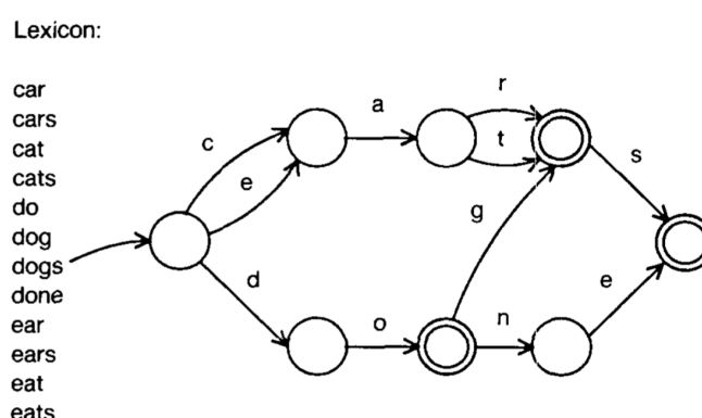
FIGURE 6 – Exemple d'une structure DAWG. (Source : [1])
