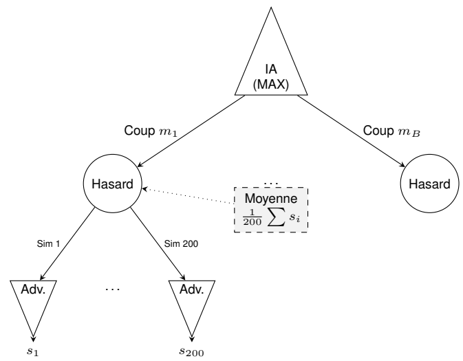
FIGURE 4 – Agrégation Probabiliste
