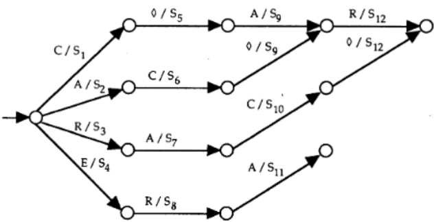
FIGURE 7 – Graphe du GADDAG semi-minimisé pour « CARE ». (Source : [7])
