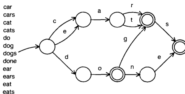
FIGURE 6 – Exemple d'une structure DAWG. (Source : [2])
