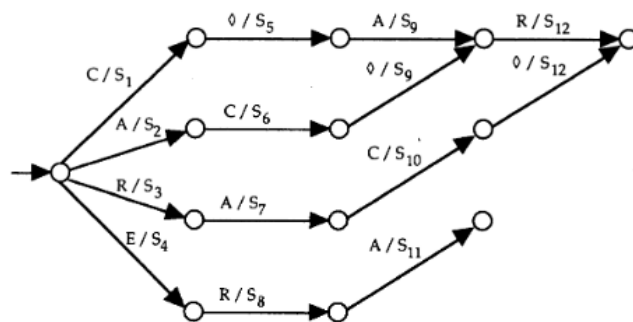
FIGURE 7 – Graphe du GADDAG semi-minimisé pour « CARE ». (Source : [8])
