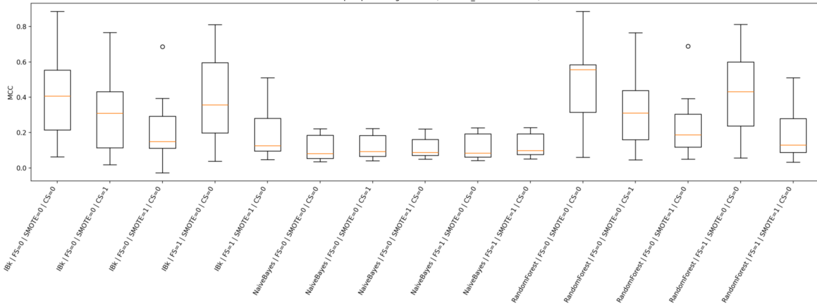
MCC boxplot per configurazione (da weka_walkforward.csv)
