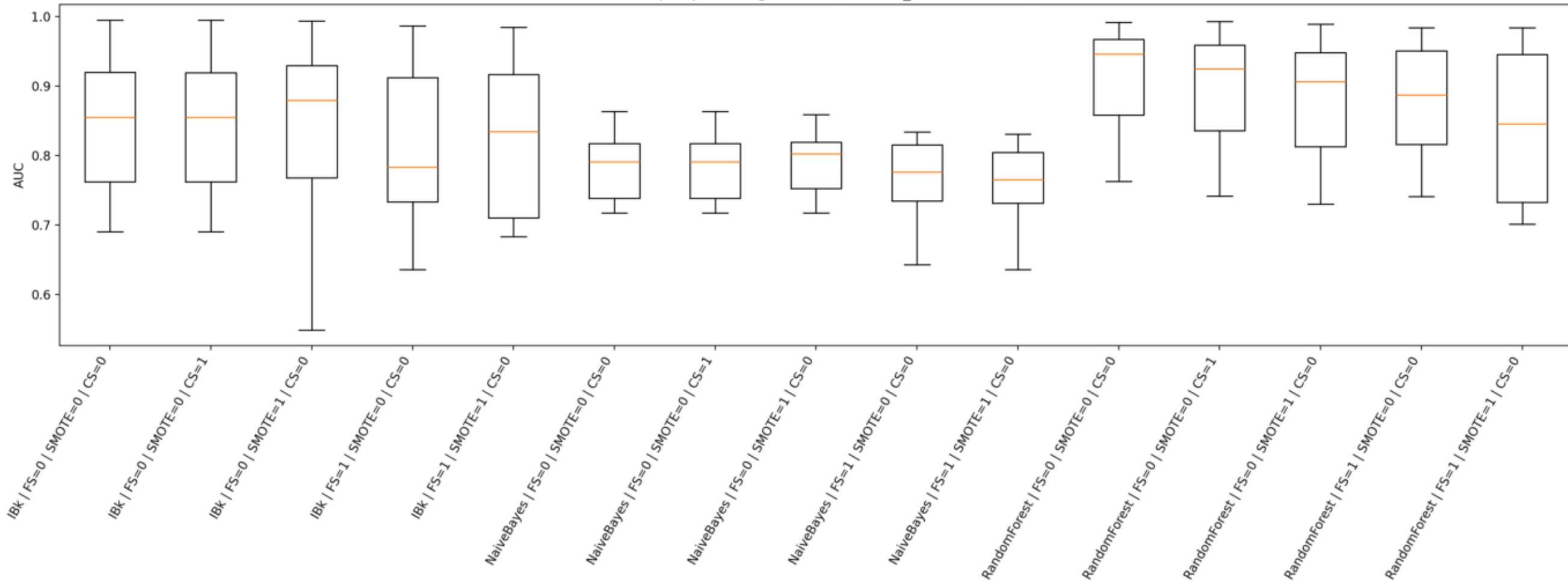
AUC boxplot per configurazione (da weka_walkforward.csv)
