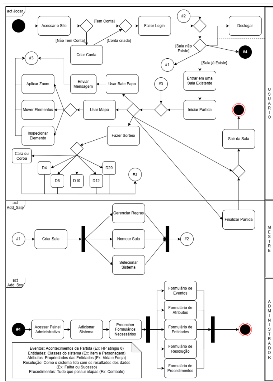
Figura 2 – Diagrama de atividades.
