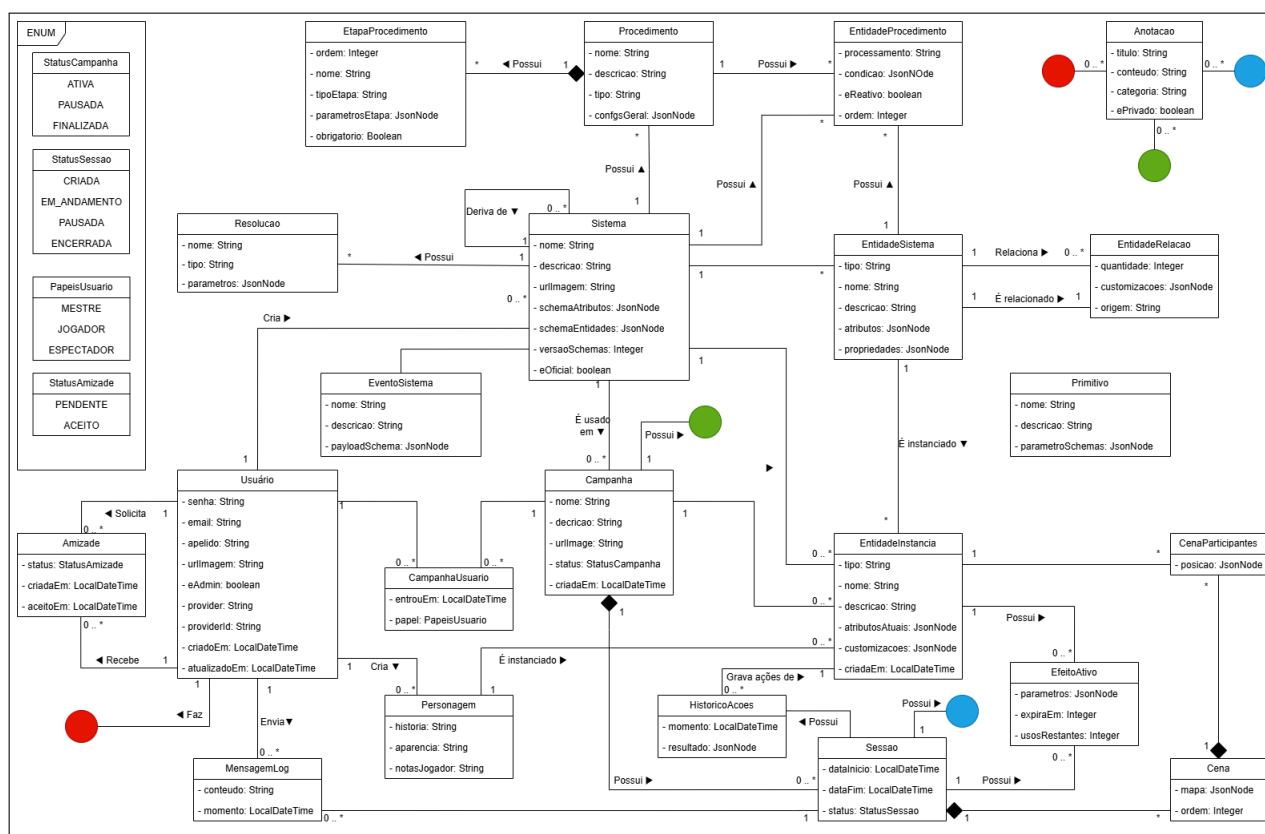
Figura 3 – Diagrama de Classes de Domínio
