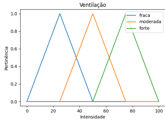
Fig. 4. Funções de pertinência triangulares para a variável ventilação (saída) .
