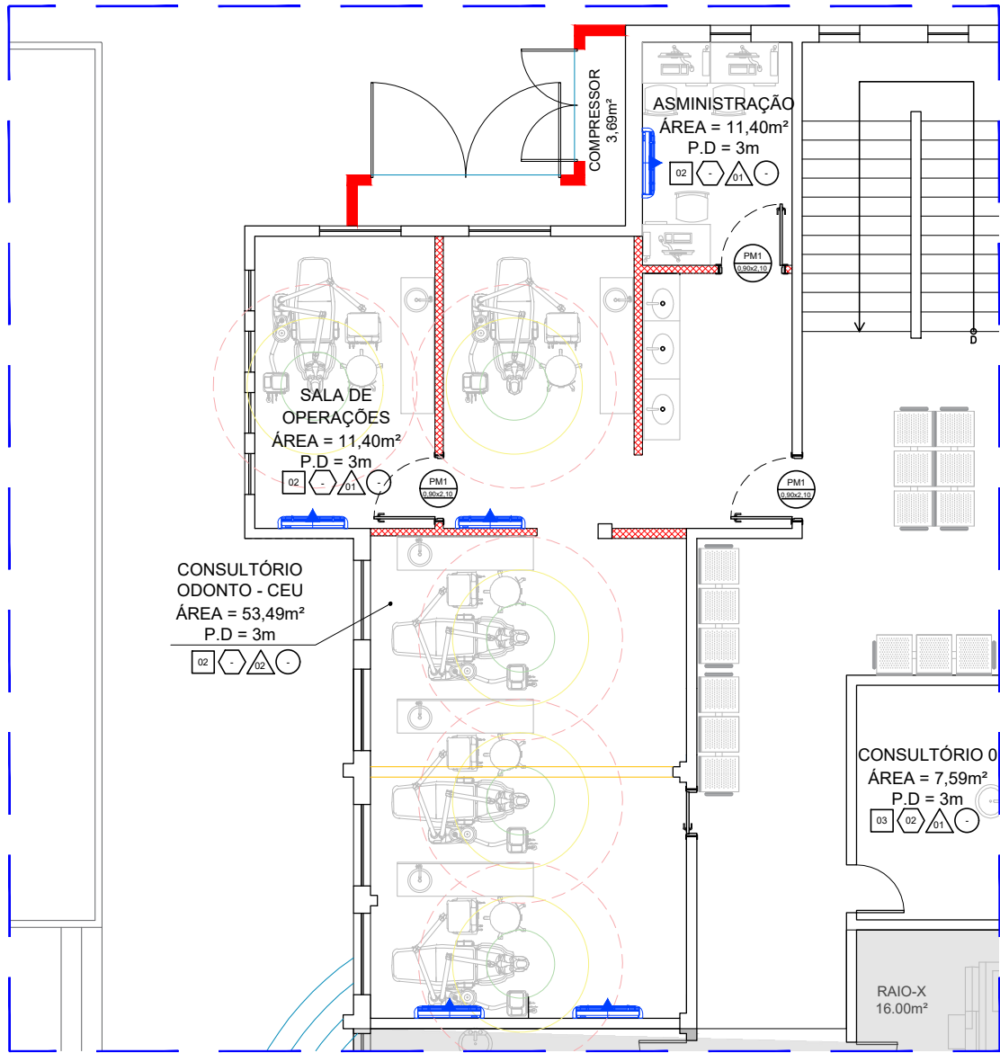
01 PLANTA TETO ESCALA 1/100
