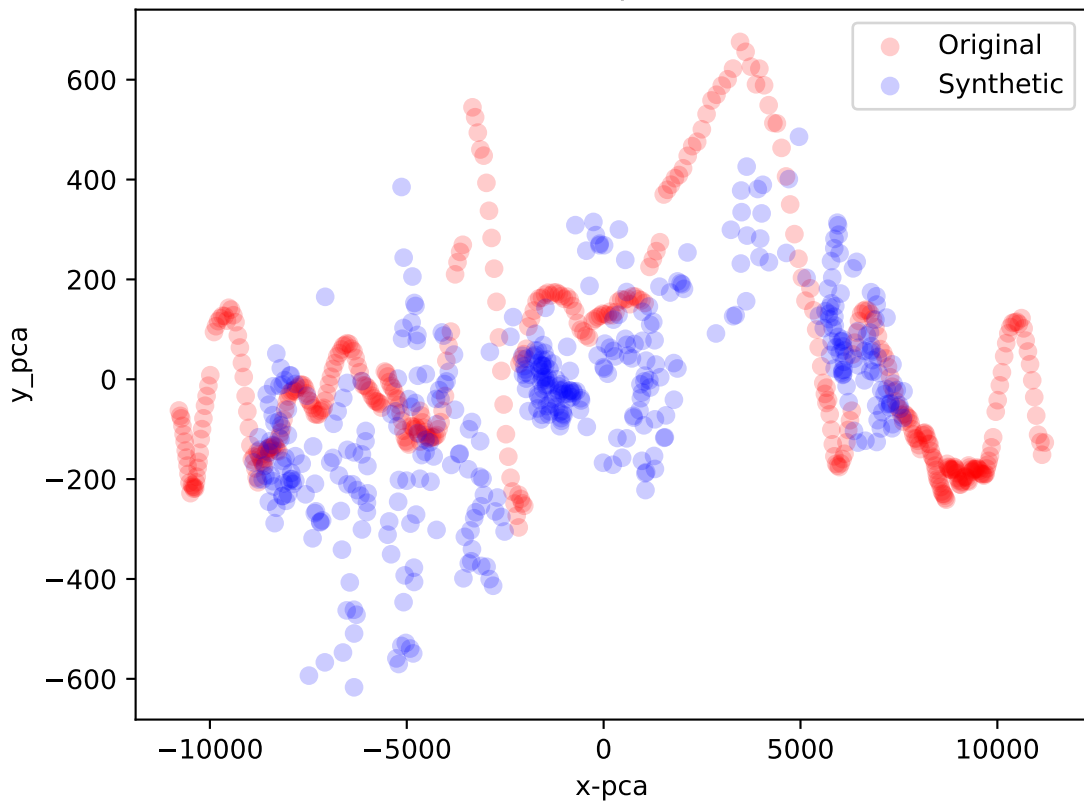
PCA plot
