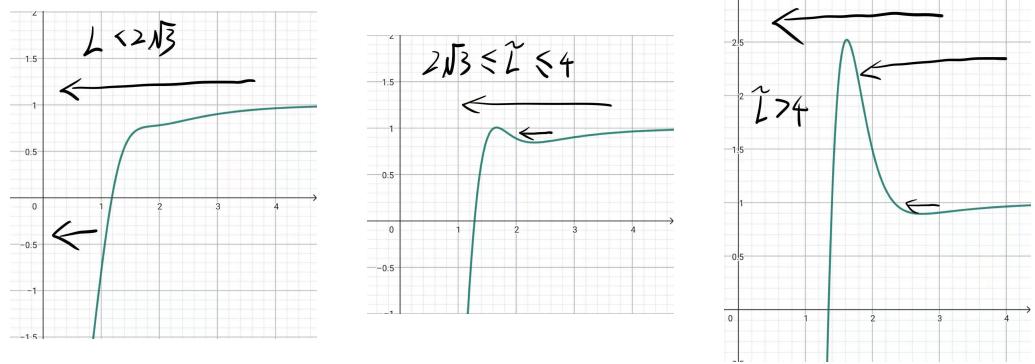
图 3: 爱因斯坦引力散射
