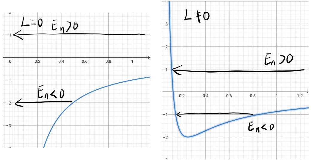
图 2: 牛顿引力散射
