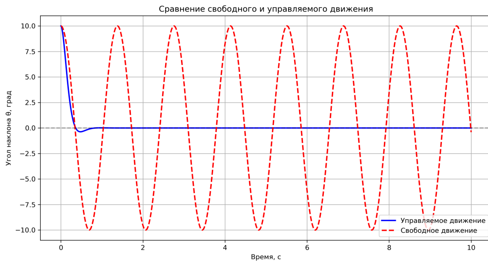
Рисунок 4 — Сравнение свободного и управляемого движения
