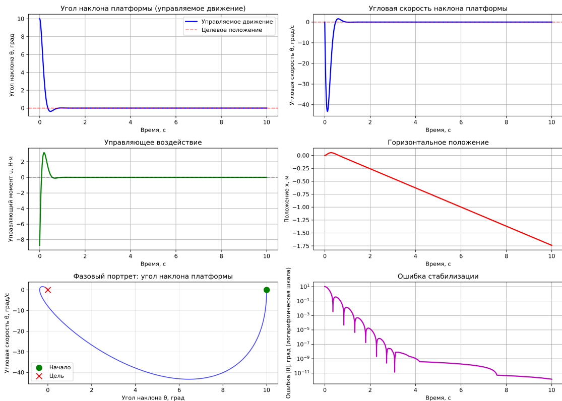
Рисунок 3 — Динамика управляемого движения Segway с контроллером по выходу
