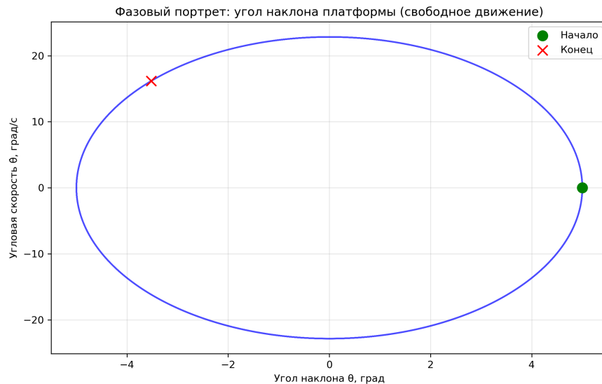
Рисунок 2 — Фазовый портрет свободного движения
