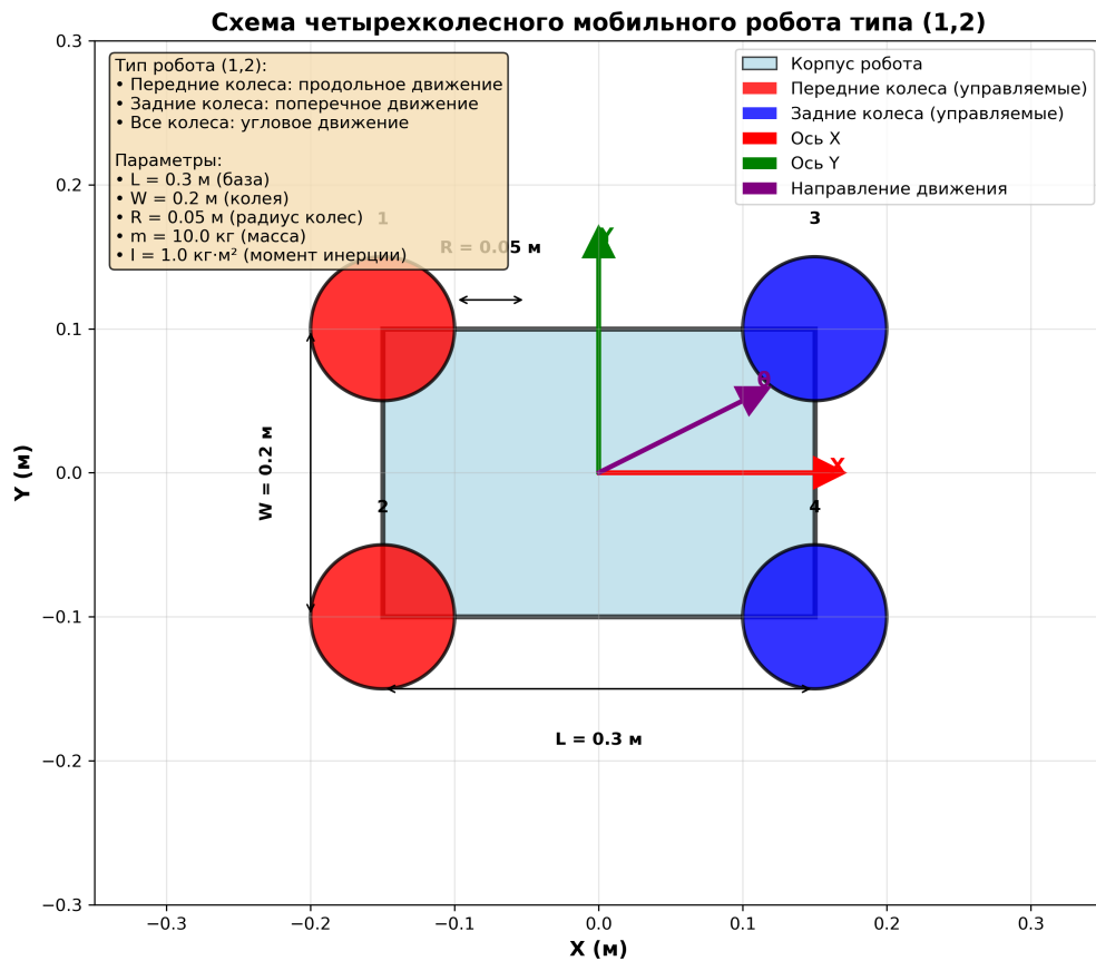
Рисунок 2 — Схема четырехколесного мобильного робота типа (1,2)
