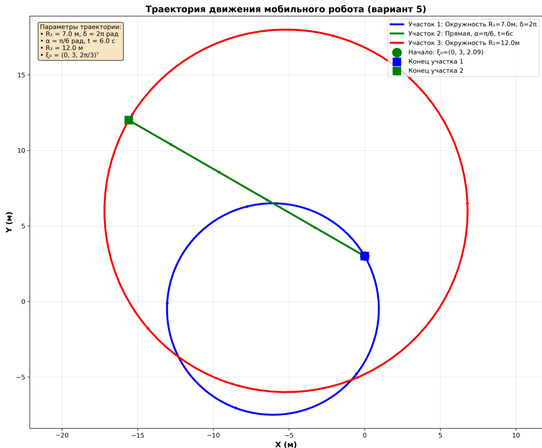
Рисунок 3 — Траектория движения мобильного робота (вариант 5)
