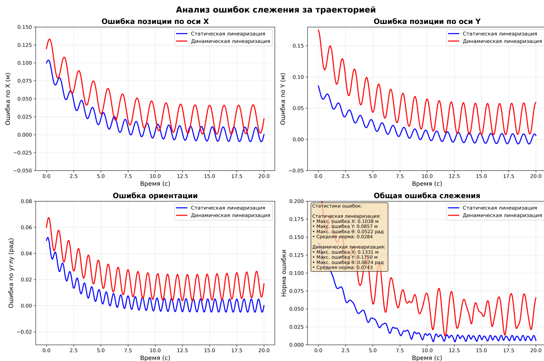
Рисунок 5 — Анализ ошибок слежения за траекторией
