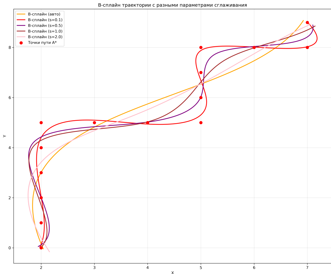
Рисунок 5 — B-сплайн траектории с разными параметрами сглаживания
