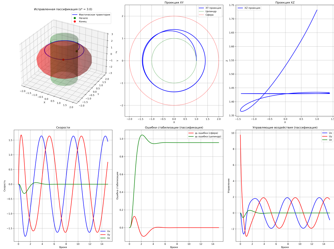
Рисунок 5 — Лучший результат стабилизации 3D траекторий методом пассивфикации ( s^* = 3 )
