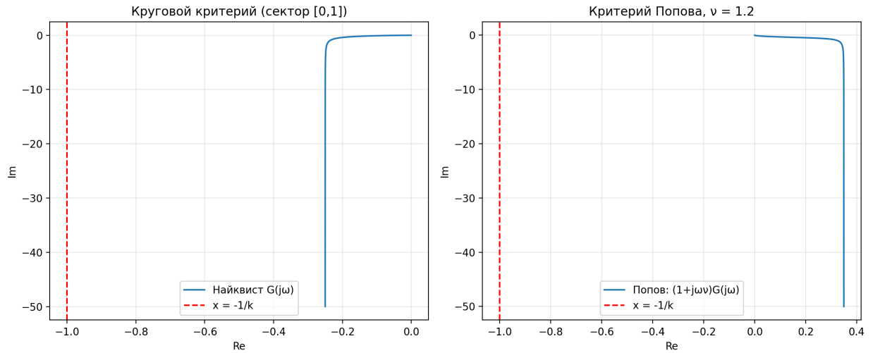
Рисунок 2 — Найквист и кривая Попова для G(s) = 1/(s(s+2)) , сектор [0,1]
