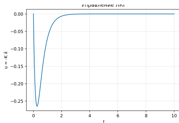
(б) Управление u = -K\hat{x}
