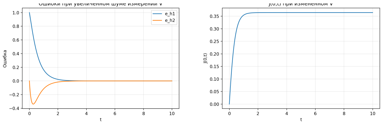
(а) Ошибки при V_{\text{mod}}
