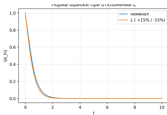
(а) Нормы ошибки вектора e_h
