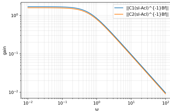
(в) Оценка H_\infty -норм передаточных функций
