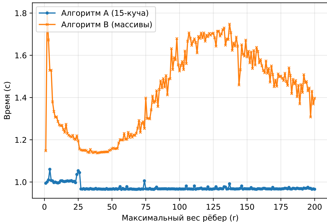
Плотный граф ( m \approx n^2 )
