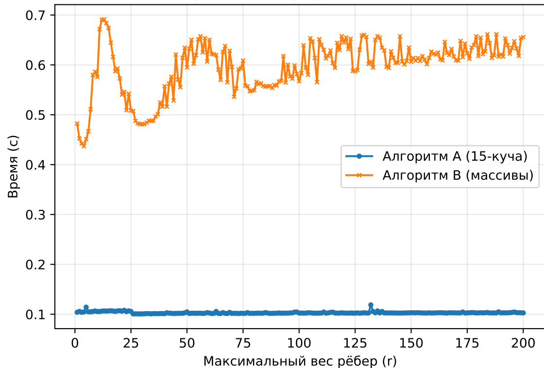
Разреженный граф ( m \approx 1000 \cdot n )
