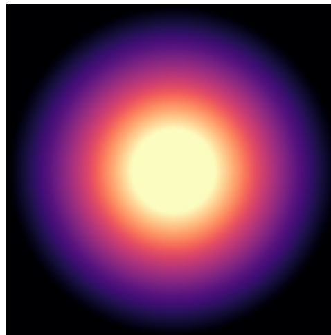
UGC01281
