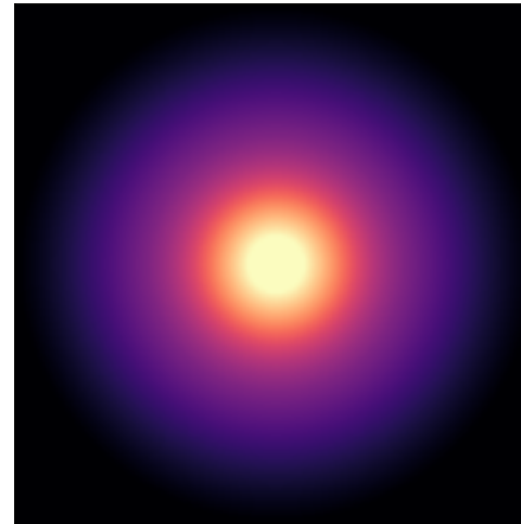
NGC3893
