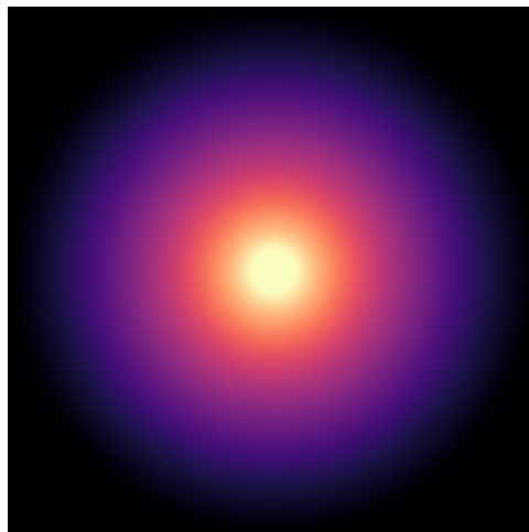
UGC05829
