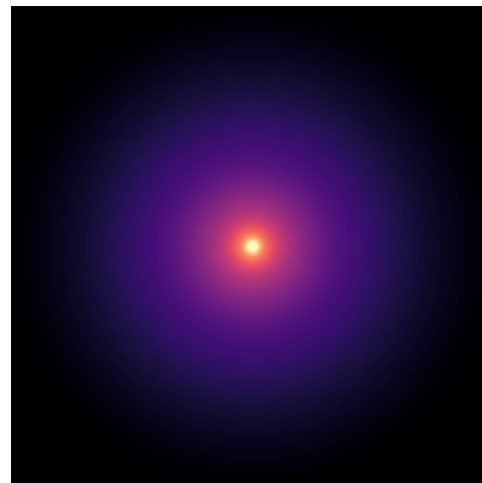
UGC06930
