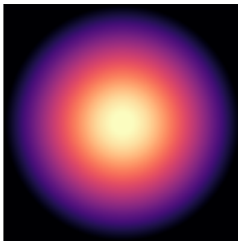
NGC0055
