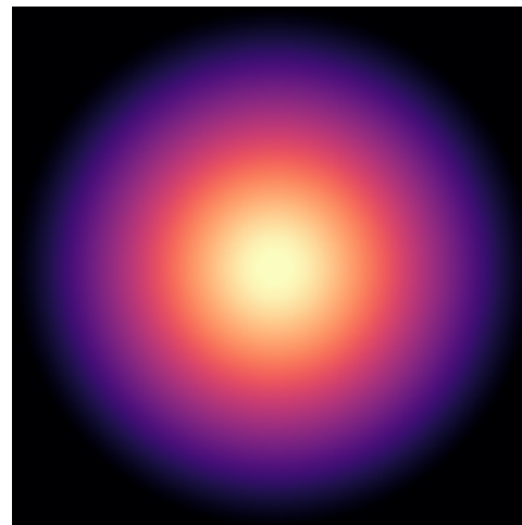
DDO168
