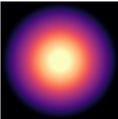
UGC05764
