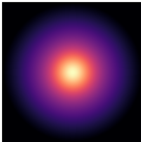
F568-V1
