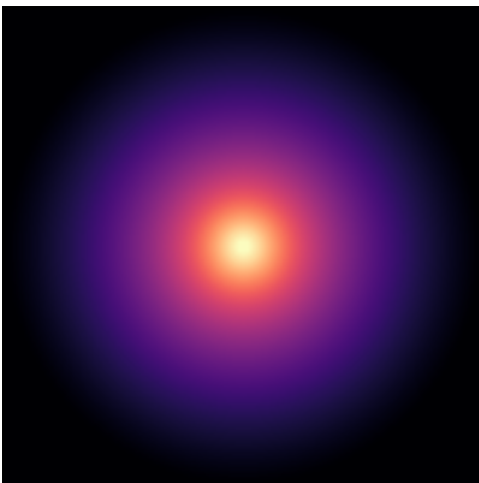
UGC00891
