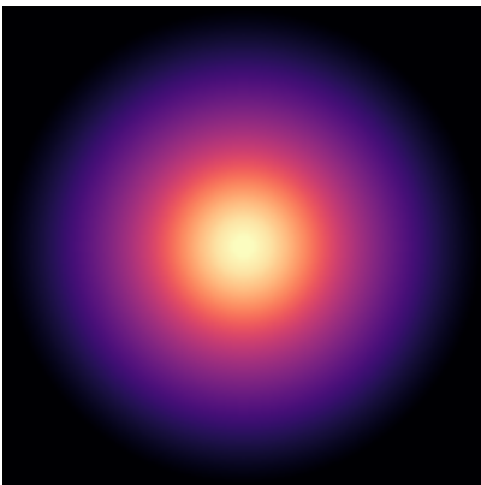
F583-4
