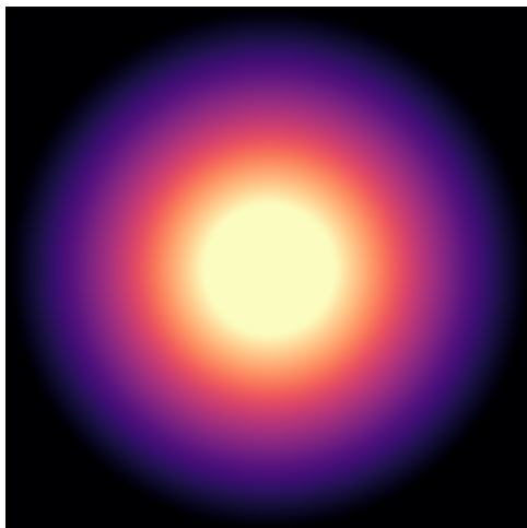
DDO154
