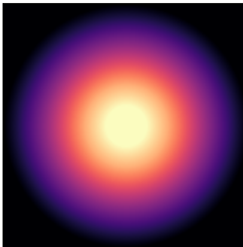
DDO161
