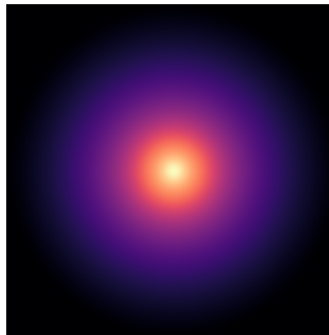
UGC05918
