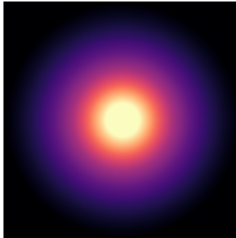
UGC07690
