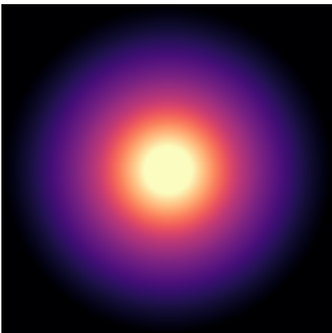
UGC06818
