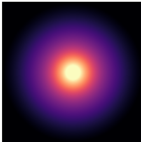
NGC6674
