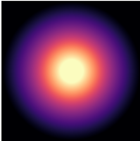
UGC06983
