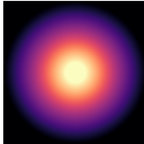
UGC07866
