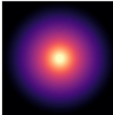
UGC06446
