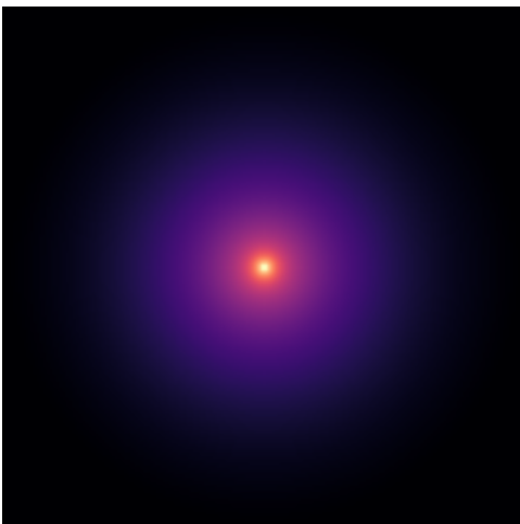
UGC03580
