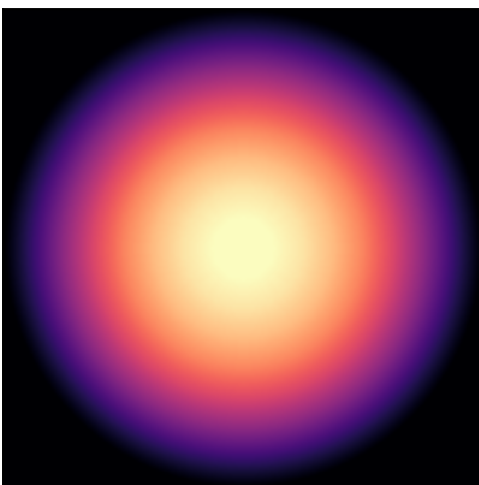
UGC10310
