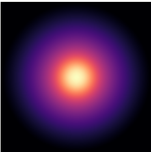
F563-V2
