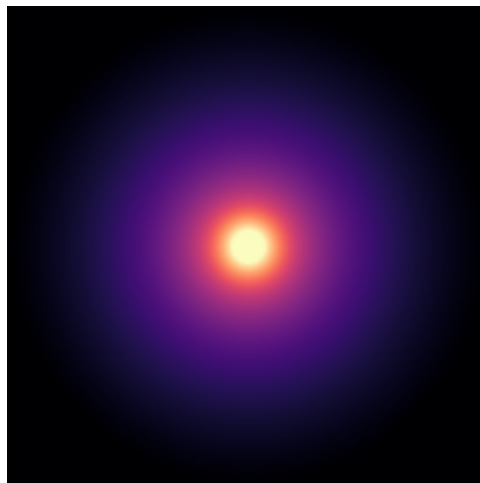
UGC04278
