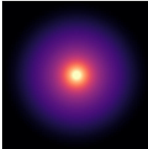
NGC3769
