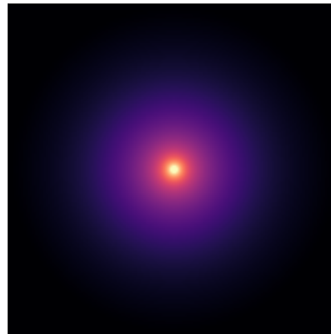
UGC05253
