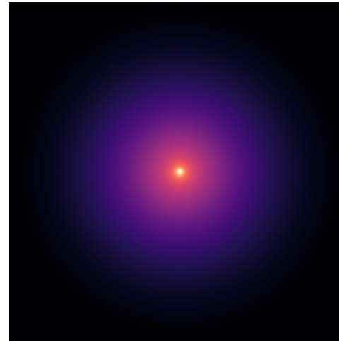
PGC51017
