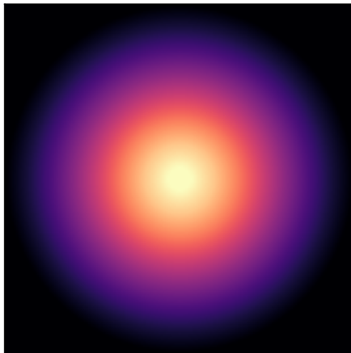
UGCA442
