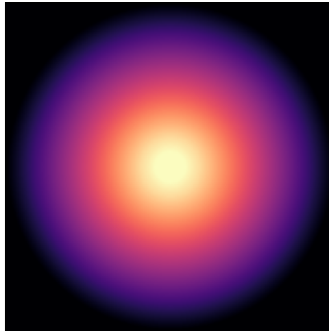
UGC06399
