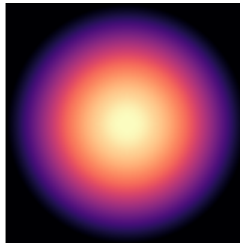
NGC3521
