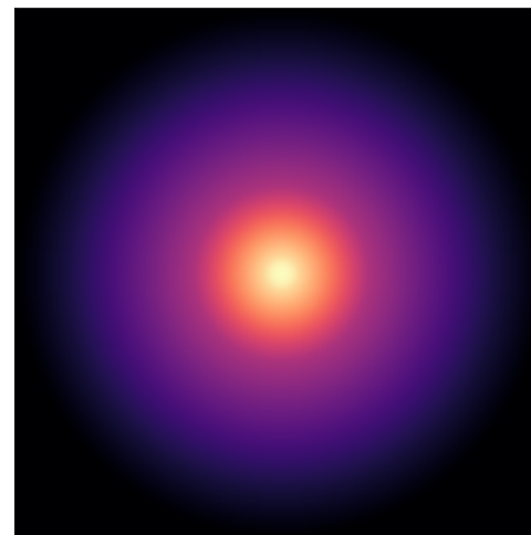
UGC11820
