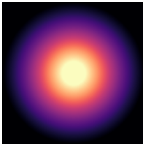
F565-V2
