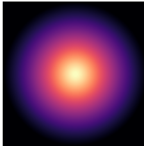
UGC05005
