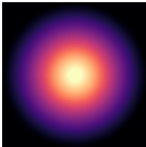
NGC0055
