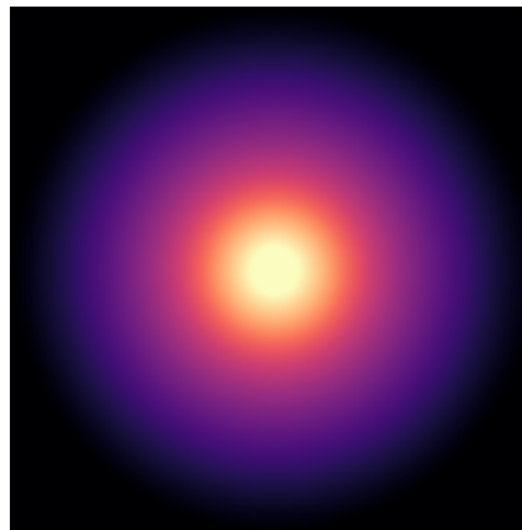
UGC09133
