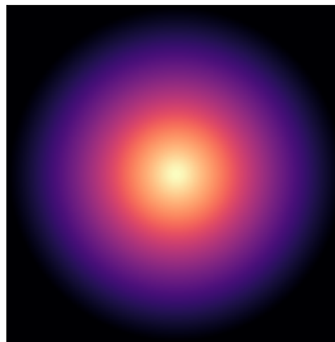
F571-8
