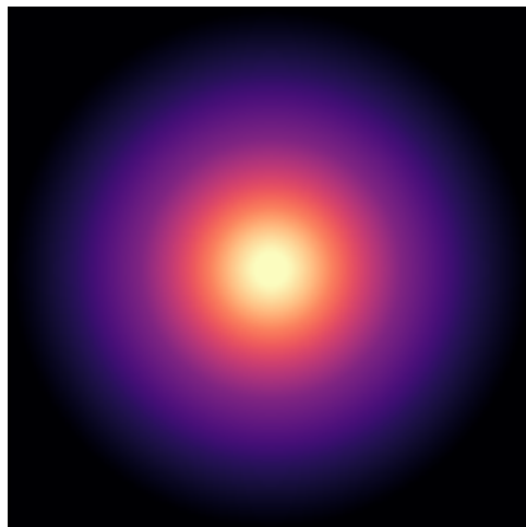
UGC01230
