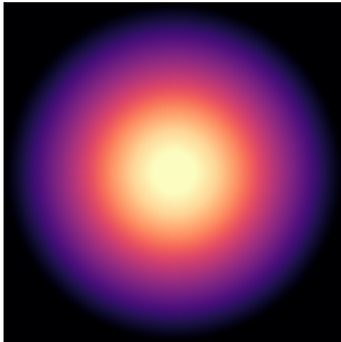
UGC07608
