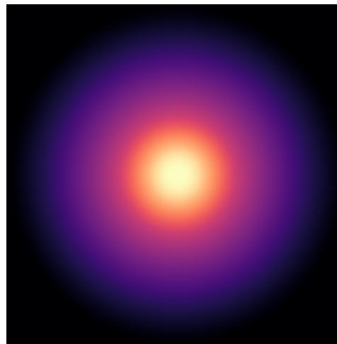
F567-2
