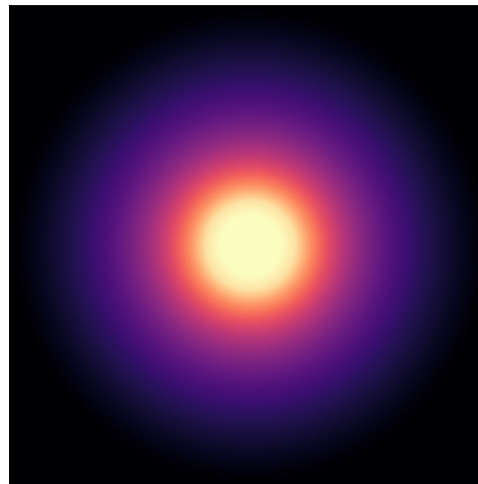
UGC02487
