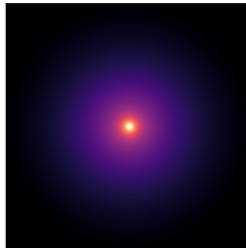
UGC04325
