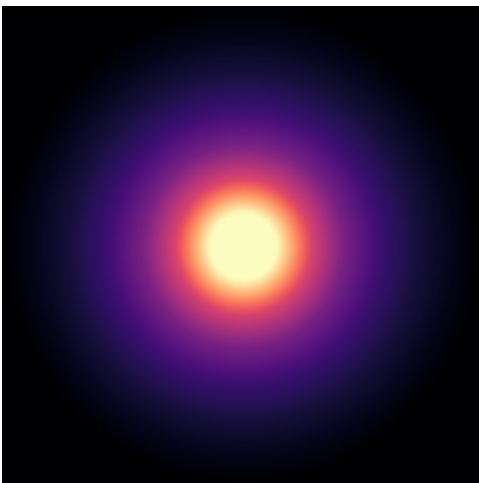
NGC4217
