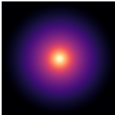
UGC09037
