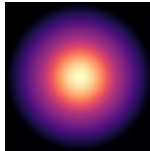
UGC05986
