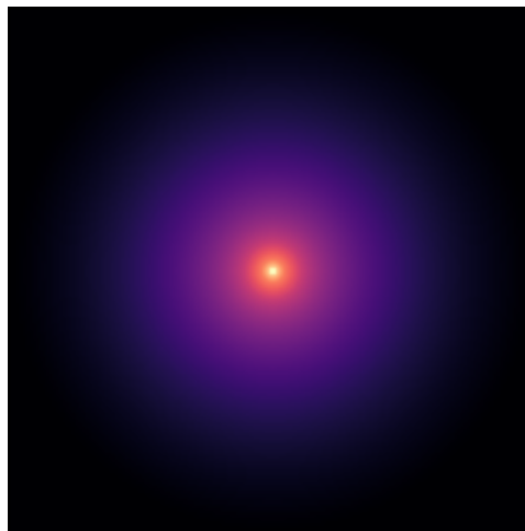
UGC06923
