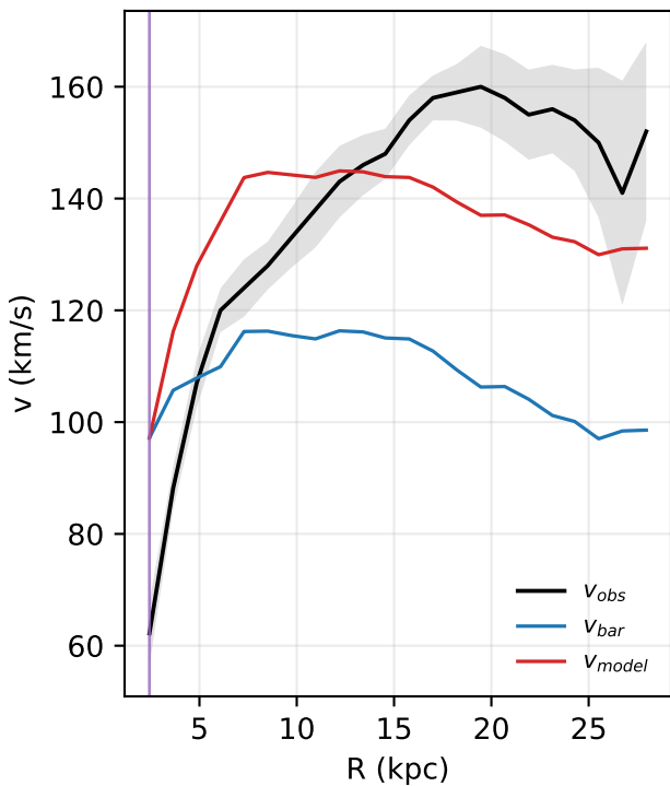
UGC09037: rotation curve
