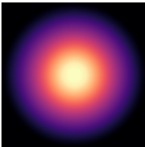
ESO079-G014
