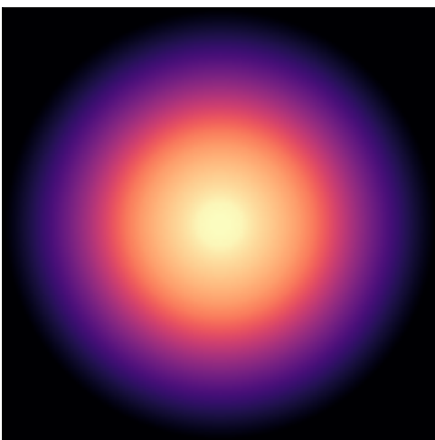
DDO170
