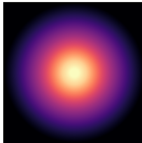
ESO444-G084
