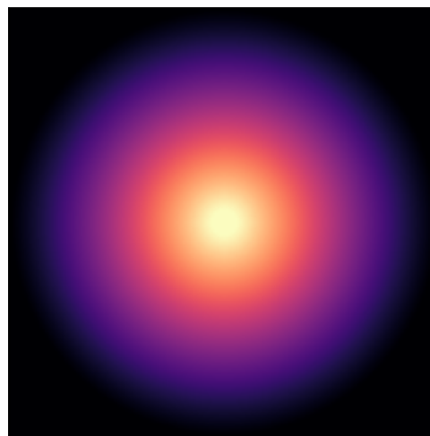
ESO116-G012
