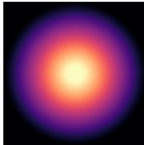
DDO168
