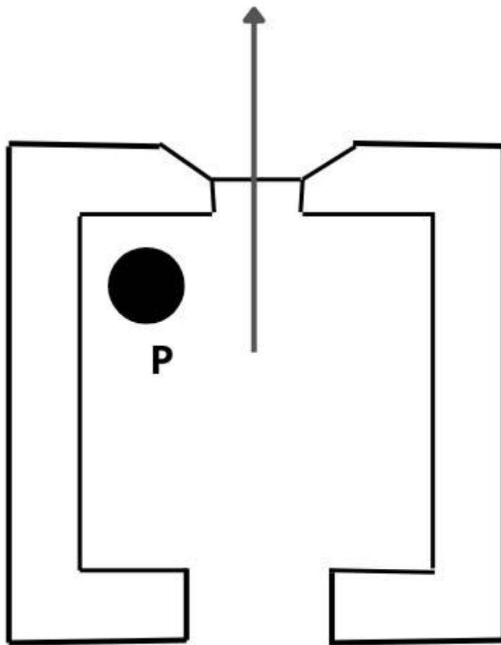
Version frontale du pillbox (nous pouvons voir l'emplacement du périscopie sur le schéma)
