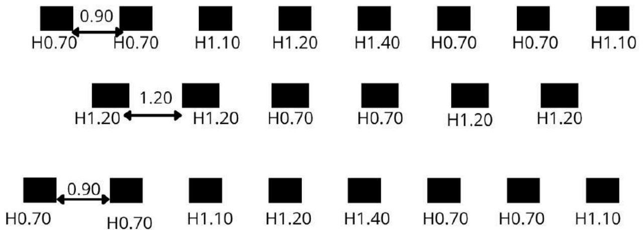
Schéma d'implantation des rails antichars.
