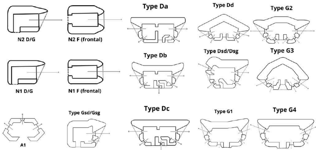
Plans types des blockhaus de la première région militaire construits dans le SFL.
