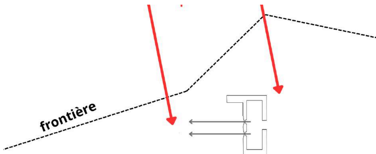
Oreillon d'un blockhaus anglais de flanquement.
