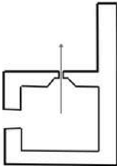
Plan d'un pillbox simple pour FM ou mitrailleuse.
