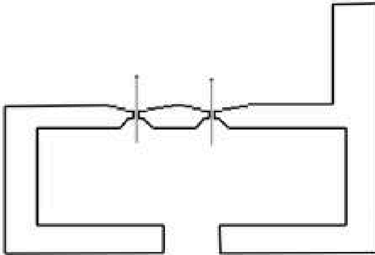
Plan d'un pillbox pour FM ou mitrailleuse avec un oreillon de flanquement.
