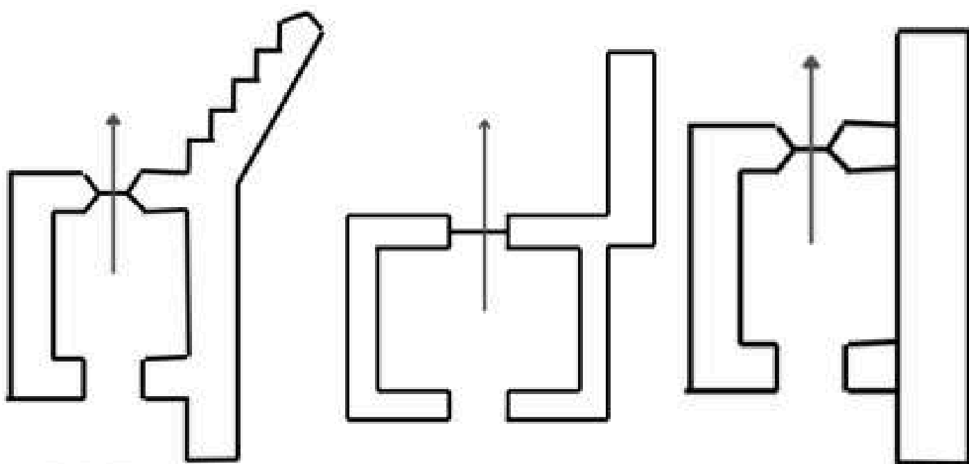
Plan des différents oreillons pour les blockhaus pour canon. Plans des types de Pillboxes. (Les noms ne sont pas basés sur des documents officiels.)
