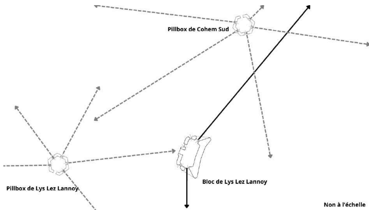
Plan de feu du Pillbox de Cohem Sud, Pillbox de Lys Lez Lannoy et Bloc de Lys Lez Lannoy (non à l'échelle).
