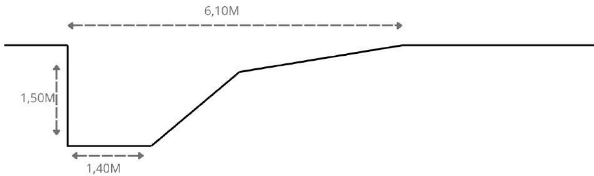
Schéma d'un fossé antichars Français.
