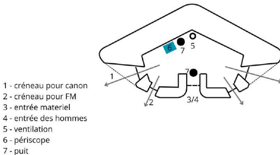
Schéma du bloc
