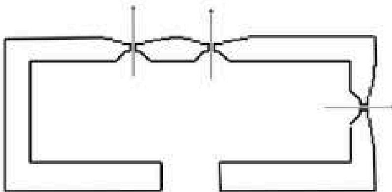
Plan d'un pillbox rectangulaire pour FM ou mitrailleuse.
