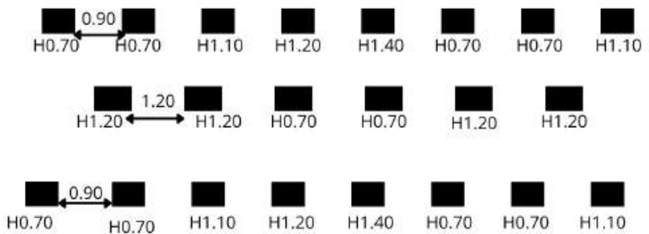
Schéma d'implantation des rails antichars.
