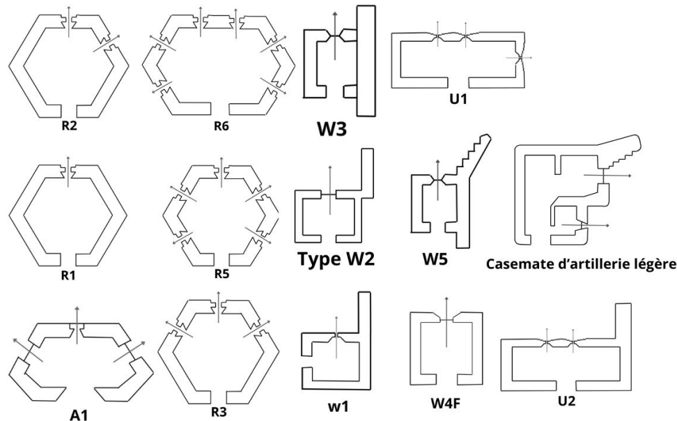
plans des Pillboxes de la B.E.F ©les blockhaus lyssois
