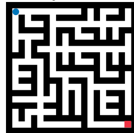
Algoritma Prim
