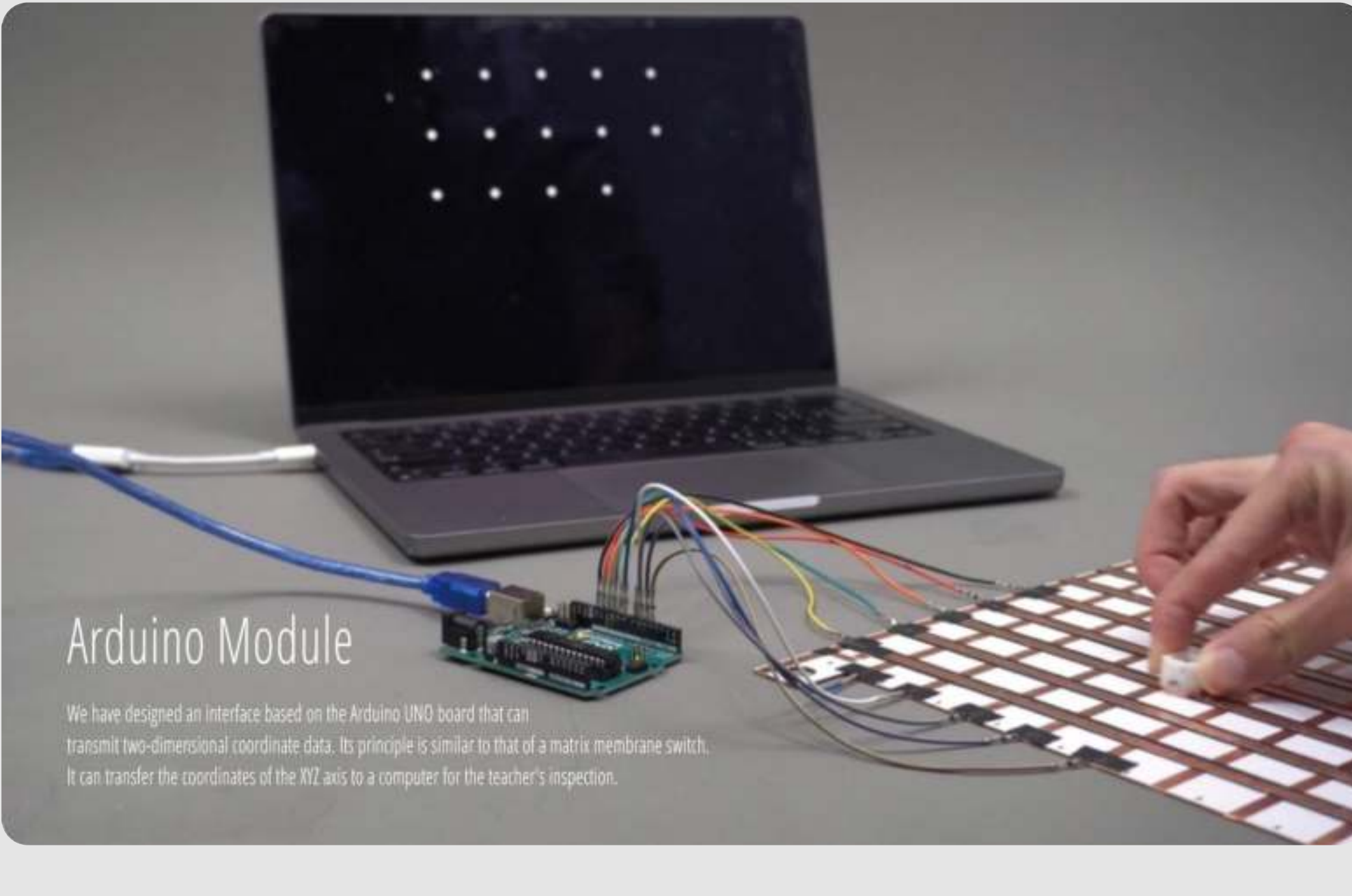
Arduino Module
