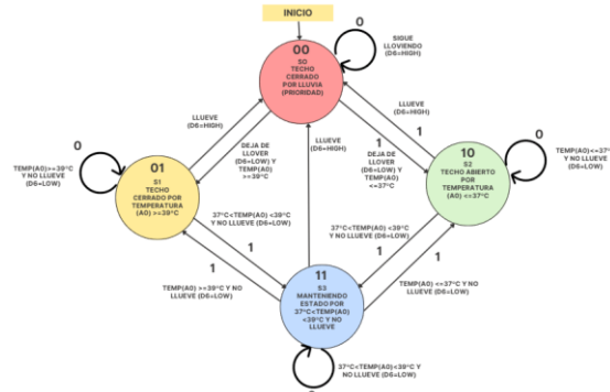
Fig. 3 Representación del grafo de estados de la máquina de estados finita.
