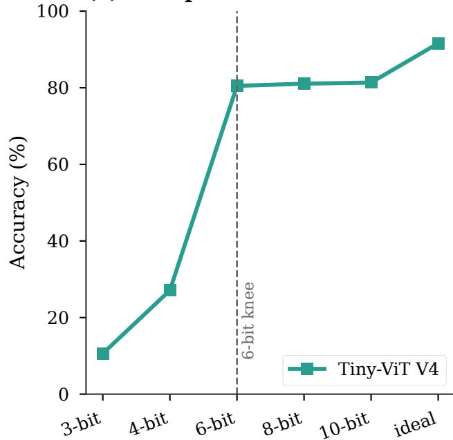
(b) ADC precision
