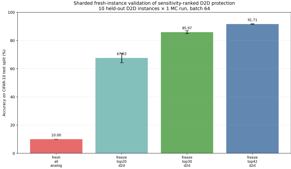
图 7.3: 基于 full42 排序的分片式 fresh-instance 保护复核。每个策略在完整 CIFAR-10 测试集上评估 10 个未见 D2D 实例、每实例 1 次 C2C 蒙特卡洛前向传播。top-30 保护在多实例上达到 85.97 \pm 1.02\% ，显著高于全新失配配置的 10.00 \pm 0.00\% ，但该图仍不是最终多次蒙特卡洛前向传播的部署协议。
