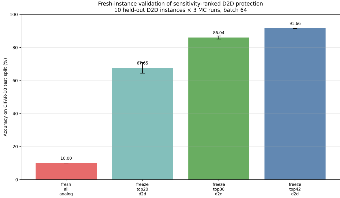
图 7.3: 基于 full42 排序的分片式 fresh-instance 保护复核。每个策略在完整 CIFAR-10 测试集上评估 10 个未见 D2D 实例、每实例 3 次 C2C 蒙特卡洛前向传播。top-30 保护在多实例上达到 86.04 \pm 0.95\% ，显著高于全新失配配置的 10.00 \pm 0.01\% ，但该图仍表示推理期保护诊断，而非已实现的混合精度硬件方案。
