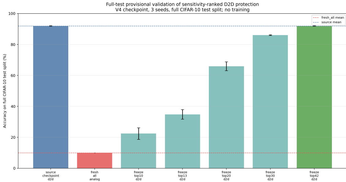
图 7.2: 基于 full42 排序的完整 CIFAR-10 测试集保护曲线。freeze_topK_d2d 将排名前 K 的敏感层保留为 checkpoint D2D, 其余层重采样为 fresh D2D。结果显示 top-30 保护可恢复到 86.06 \pm 0.23\% , 但该图仍为推理期定位诊断, 不是最终 fresh-instance 部署验证。
