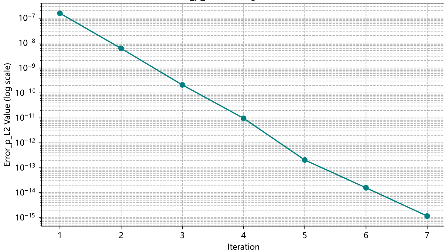
Error_p_L2 Convergence (Va=0.1)
