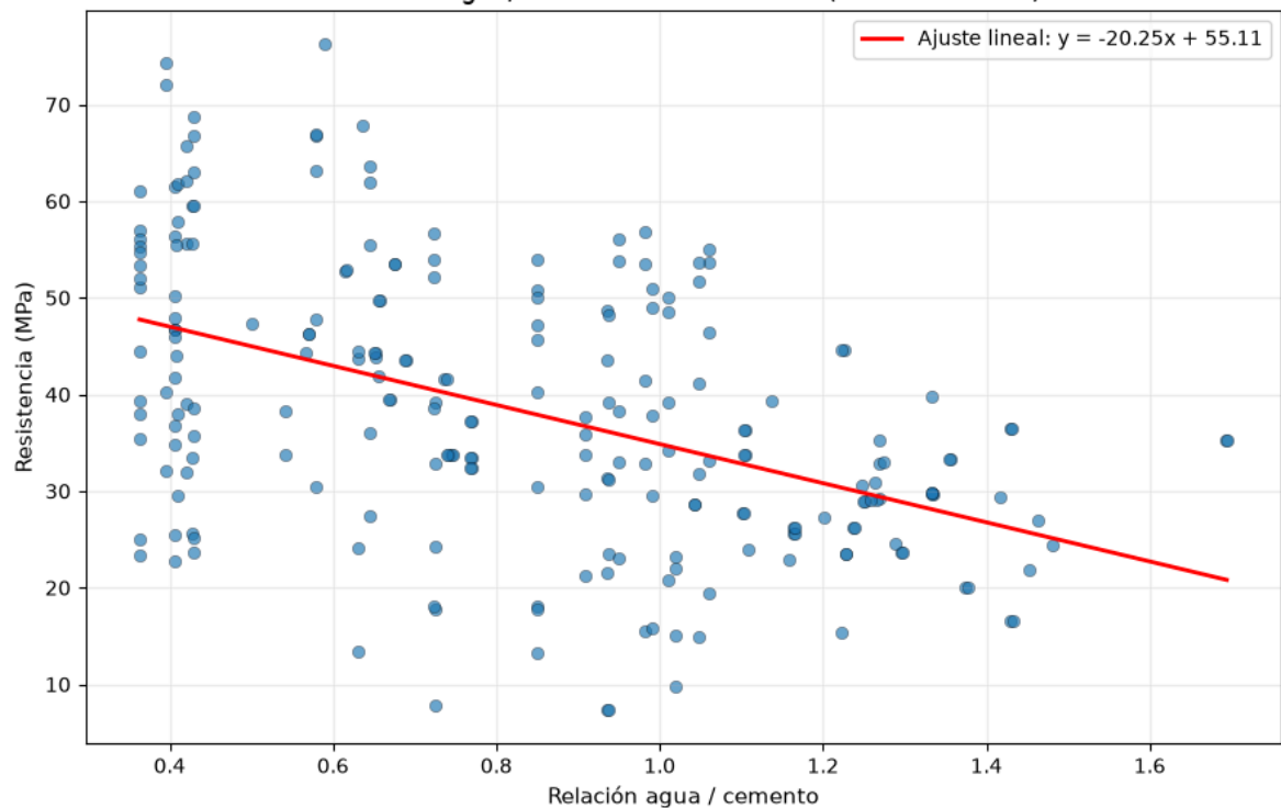
Relación agua/cemento vs resistencia (datos sin ceros)
